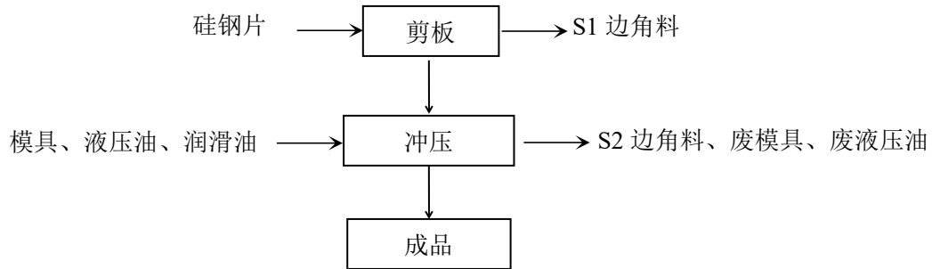
图 5-1 冲压件生产工艺流程
