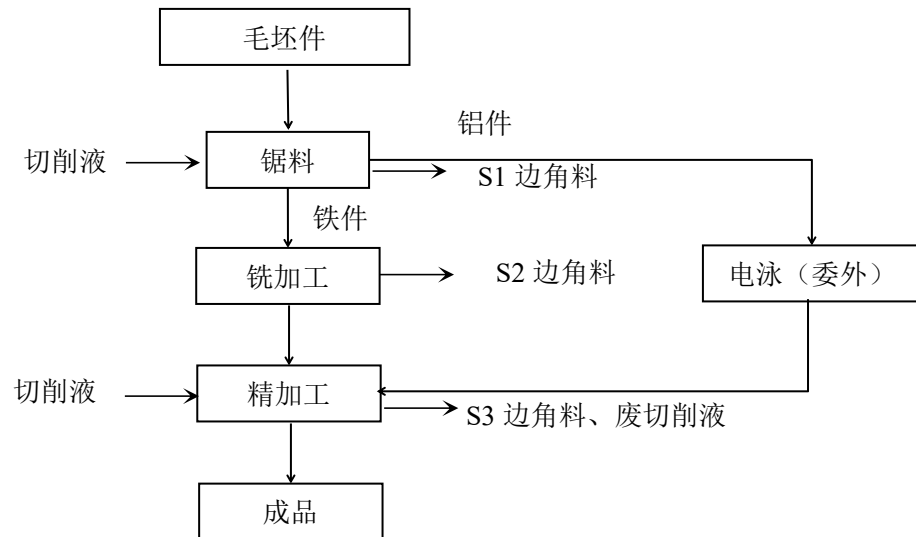
图 5-1 电机端盖生产工艺流程
